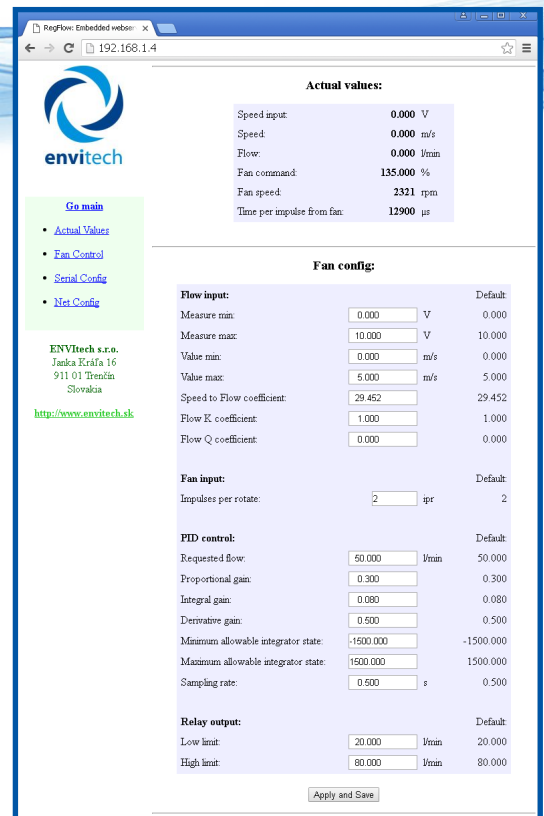
WEB stránka pre konfiguráciu regulátora
